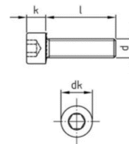
Vis M8
